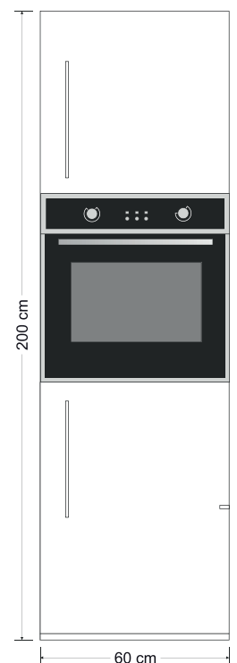
HOB - H2000
