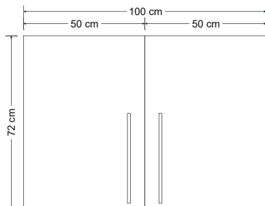
HS 100 - Skizze
