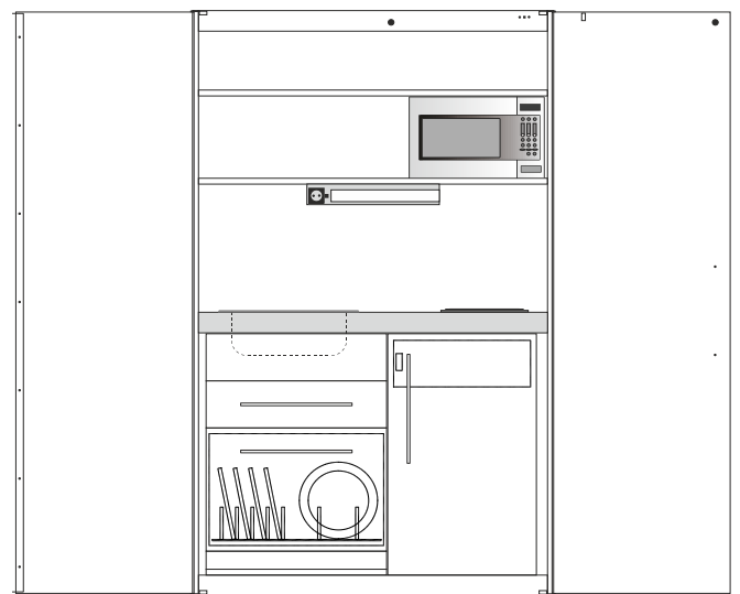
Skizze: SKM - mit Vollausrüstung
