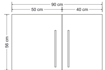
HS 90 - Skizze
